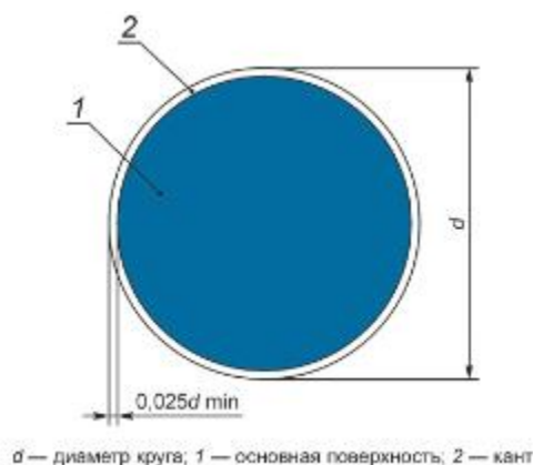
d — диаметр круга; 1 — основная поверхность; 2 — кант
