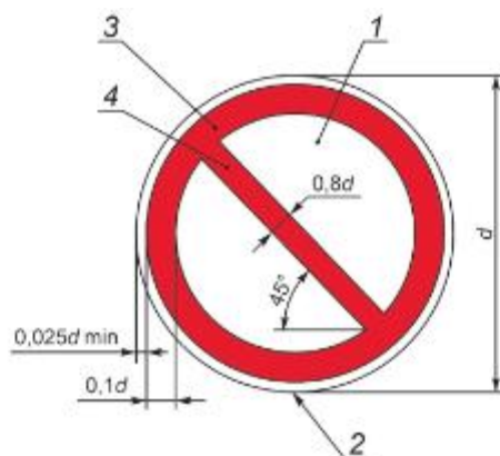
d — диаметр круга; 1 — основная поверхность; 2 — кант; 3 — кайма; 4 — поперечная полоса
